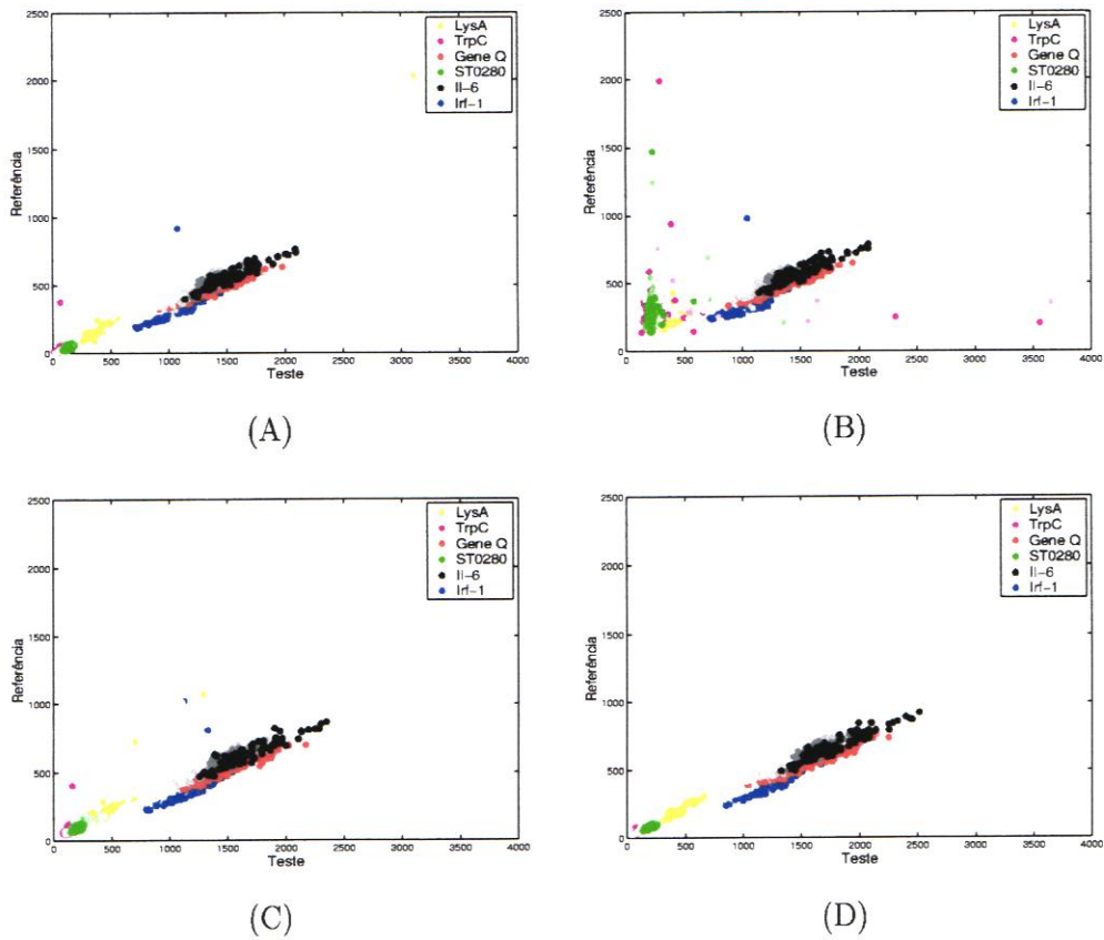
Figura 14: Scatter plots do experimento exp3/1.
