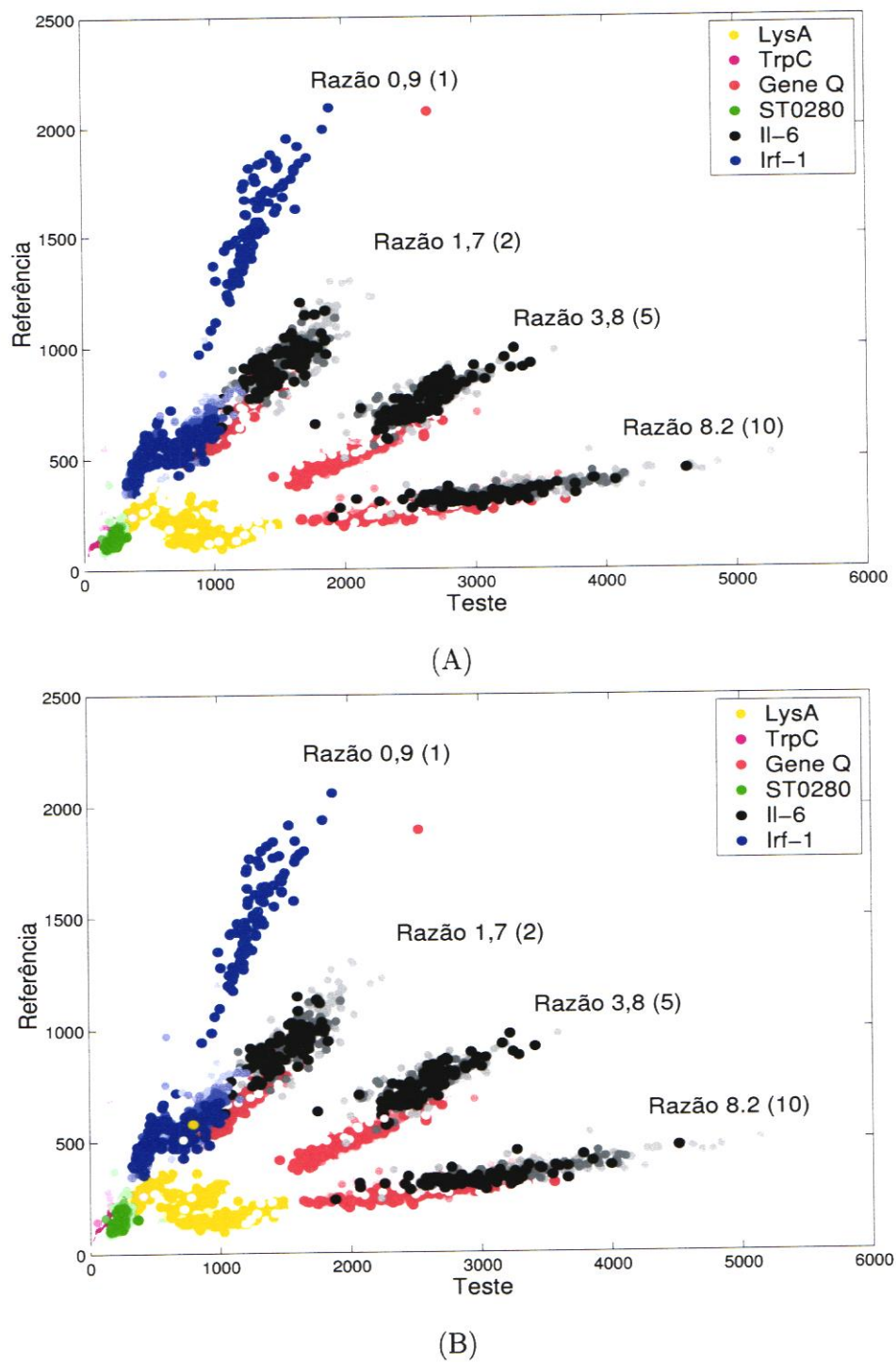
Figura 22: Validação da metodologia de cDNA microarray .
