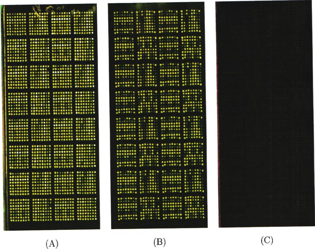
Figura 9: Comparação entre as proporções de alvo/sonda. Essa figura ilustra as diferenças observadas entre as proporções de material flutuante e fixado, com base nos experimentos 1, 2 e 3 descritos na Tabela 7. (A) - experimento 1 (500 vezes mais cDNA flutuante em relação ao fixado), (B) - experimento 2 (5 vezes mais cDNA flutuante em relação ao fixado), (C) - experimento 3 (20 vezes mais cDNA fixado em relação ao flutuante).
