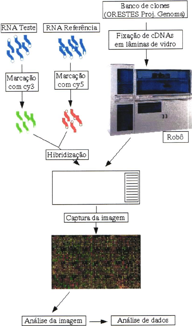
Figura 3: A metodologia de microarray .
