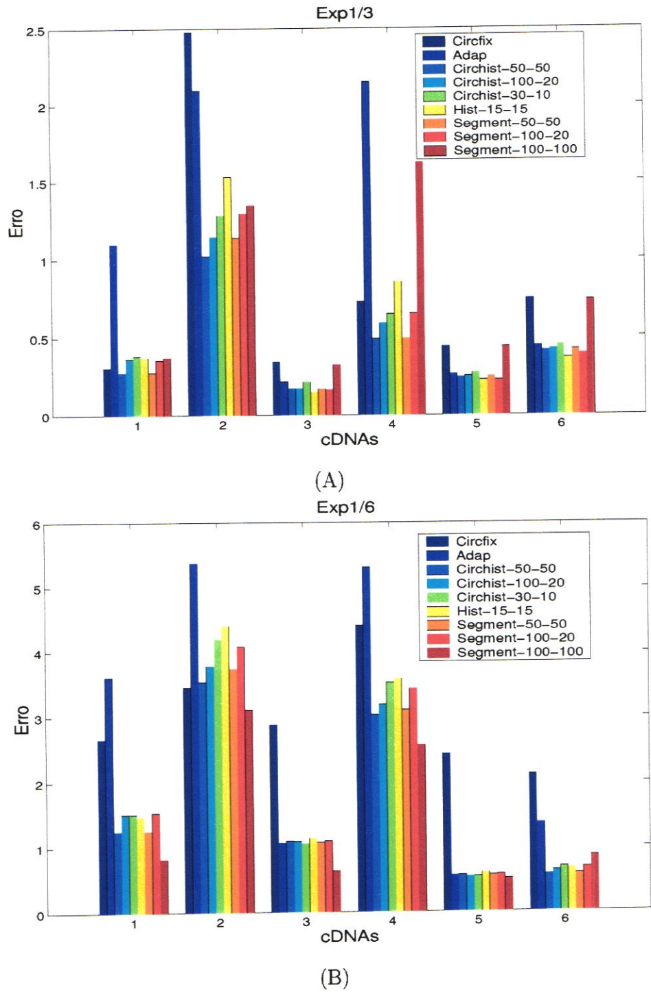
Figura 25: Erros cometidos nos experimentos exp3/1 e exp6/1.
