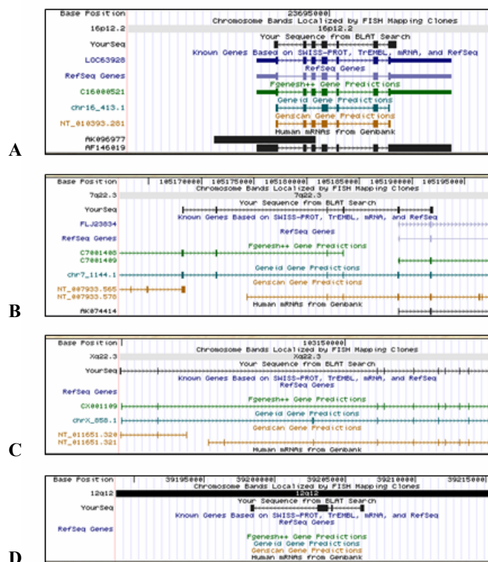
Figura 17 - Alinhamento das seqüências consensos contra a seqüência genômica. O alinhamento das seqüências consensos foi realizado contra a montagem do genoma humano disponibilizada pela UCSC utilizando o programa BLAT. As seqüências consenso estão representadas em preto (“Your sequence”), predições gênicas estão representadas em verde (“Fgenesh++”) e em areia (“GenScan”), seqüências de transcritos humanos já depositadas em bancos de dados públicos em azul (“Known genes”) e em preto (human mRNAs). (A) Seqüência consenso do TF00023 com sobreposição total com transcrito humano já conhecido. (B) Seqüência consenso do TF01102 com sobreposição parcial com transcrito humano já conhecido (C) Seqüência consenso do TF01013 sem sobreposição com transcrito humano já conhecido mas com sobreposição com predição gênica (D) Seqüência consenso do TF00125 sem sobreposição com transcrito humano já conhecido e sem sobreposição com predição gênica.
