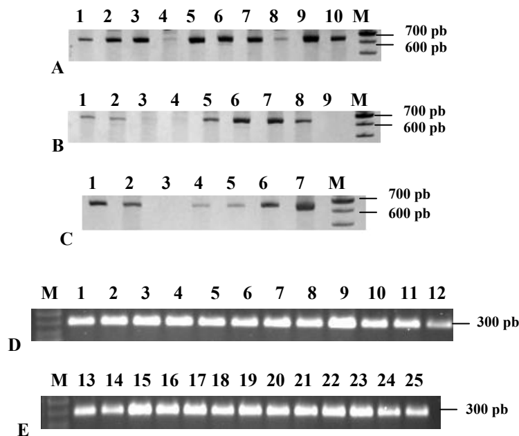
Figura 25 - Análise da expressão do transcrito C21orf100 em tumores de próstata. (A) Visualização em gel de poliacrilamida 8% da expressão do transcrito C21orf 100 em 10 amostras de tumores de próstata, (B) Visualização em gel de poliacrilamida 8% da expressão do transcrito C21orf 100 em 9 amostras de tumores de próstata, (C) Visualização em gel de poliacrilamida 8% da expressão do transcrito C21orf 100 em 6 amostras de tumores de próstata sendo a canaleta 7 referente à expressão do transcrito C21orf100 em tecido normal de próstata. (D) e (E) Visualização em gel de agarose 1% da amplificação do gene GAPDH nas amostras de cDNA dos tecidos citados anteriormente. O peso molecular (M) aplicado foi o 100bp “ladder”.
