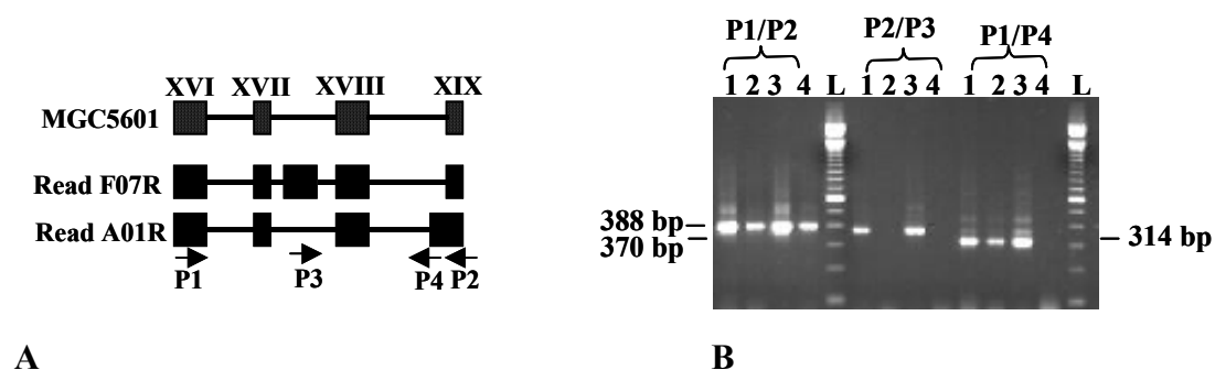
Figura 20 - Validação experimental de formas alternativas de “splicing” para o TF0200. (A) Representação esquemática do alinhamento das seqüências do TF0200 e suas respectivas ESTs com a seqüência genômica humana através do programa BLAT. Duas formas alternativas de “splicing” podem ser observadas. (B) reações de RT-PCR com iniciadores específicos para a isoforma protótipo (P1 e P2) e para as isoformas alternativas (P3 e P4). Os produtos de PCR foram analisados em gel de agarose 1,5%. Quatro tecidos distintos foram utilizados (1: glioblastoma multiforme; 2: glioblastoma; 3: carcinoma de próstata; 4: rim; L: 100bp “Ladder”).
